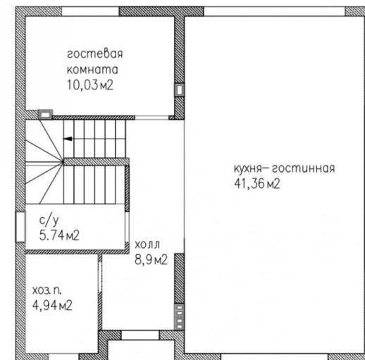
Дом 150 м² - 1 этаж
