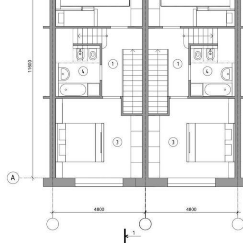
Экспликация помещений второго этажа (одна секция)
