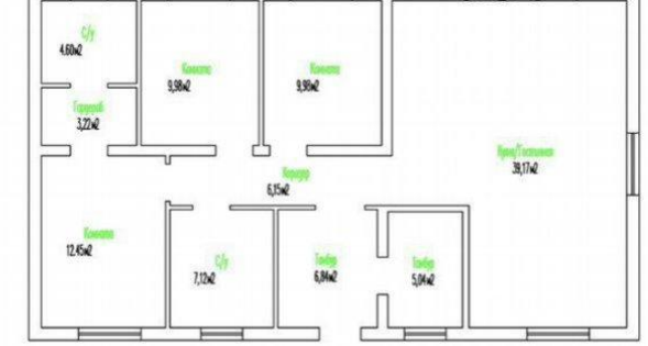
Кладочный план
