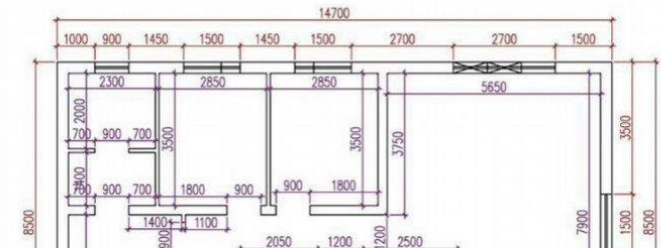
Кладочный план
