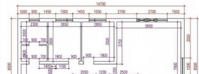
Кладочный план
