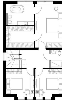
2 этаж
