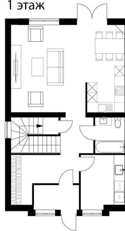
Вариант планировки №3
