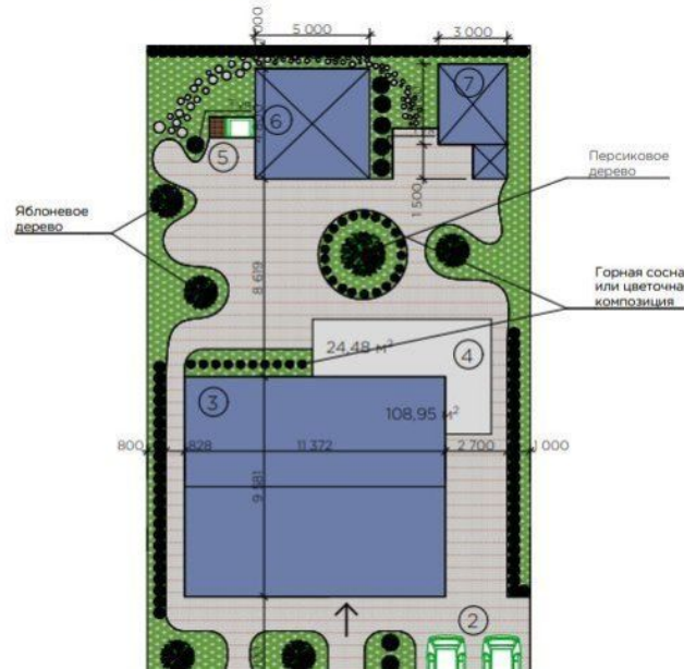
План участка с парковкой на 2 машин с изменениям
