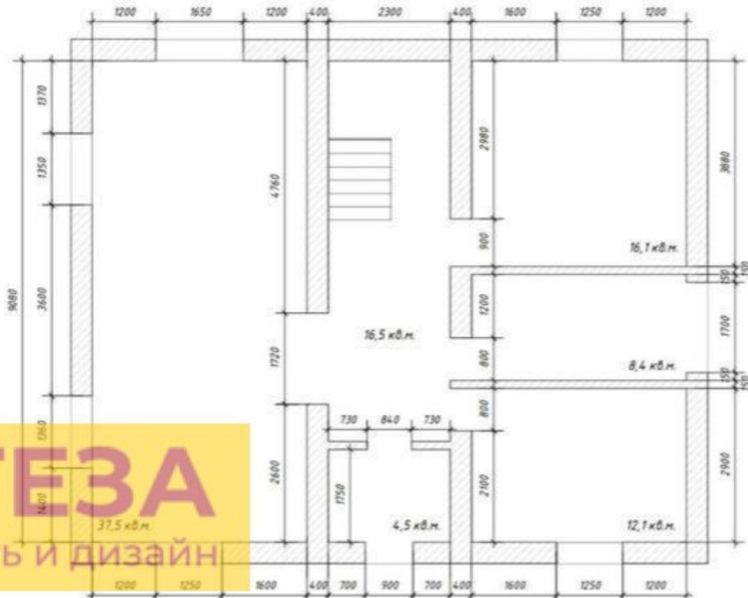
Обмерный план 1 этажа, М 1:50
