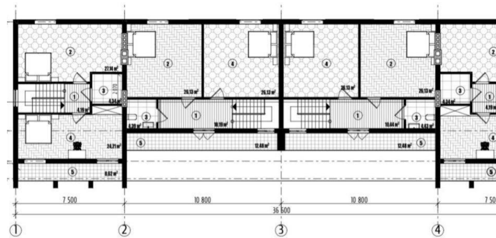
Экспликация помещений
