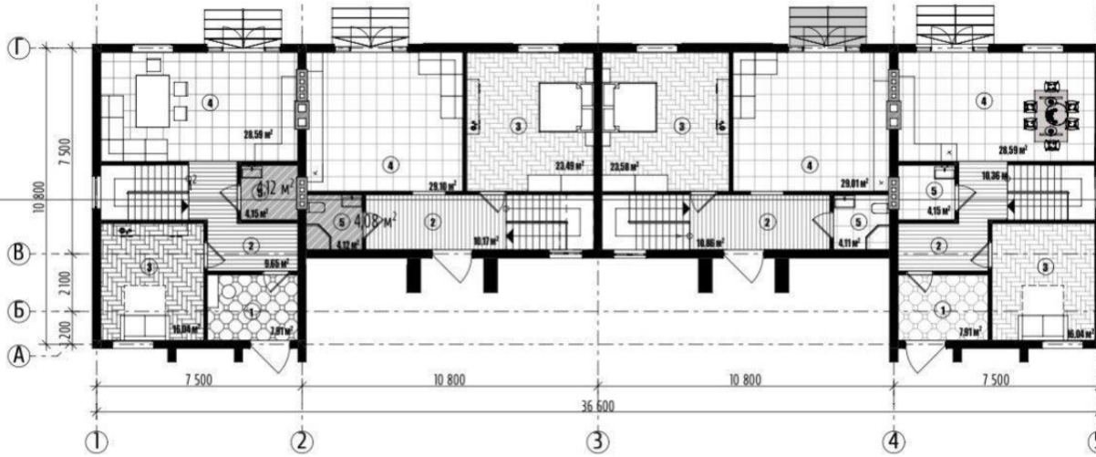
Экспликация помещений
