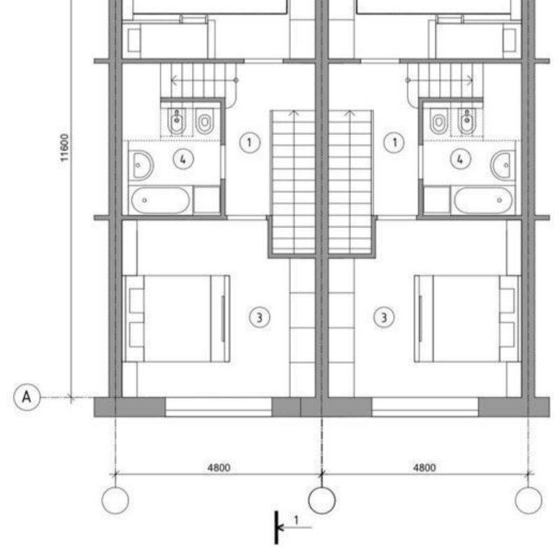
Экспликация помещений второго этажа (одна секция)
