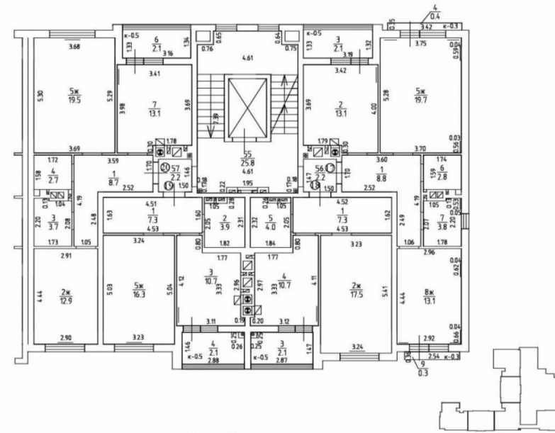
Масштаб 1:100
