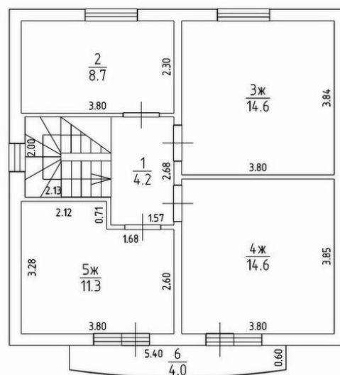
План второго этажа, Н=3,0м.
