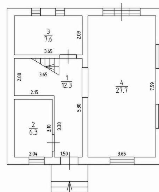
План первого этажа, Н=3,0м.
